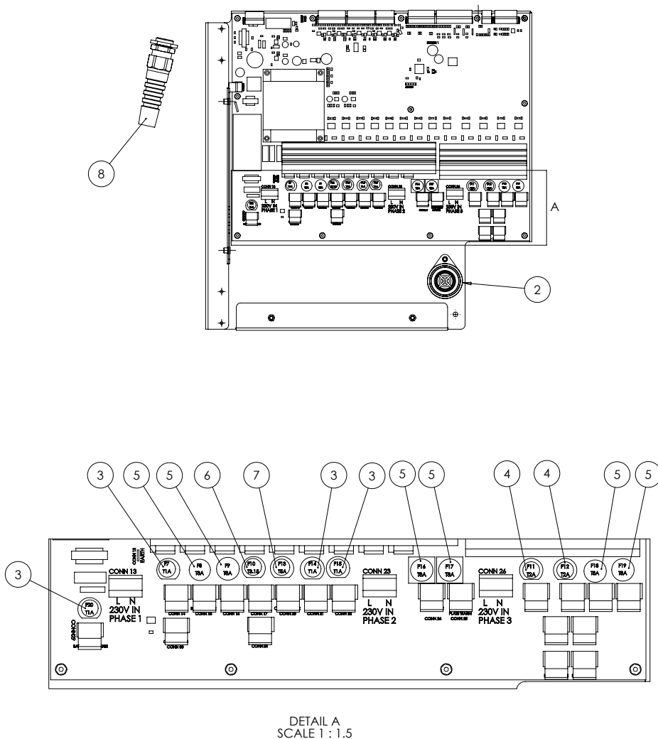
I/O BOARD DETAIL F1H, F1V, F2HR, F2VR, F2HRP
