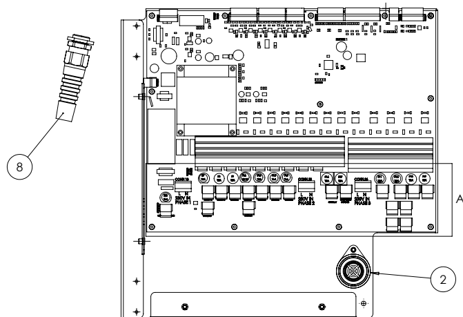
I/O BOARD DETAIL F1H, F1V, F2HR, F2VR, F2HRP
